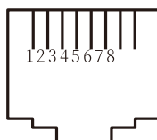
Port Modbus
